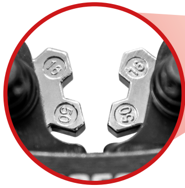
CAPACIDAD EN LA MORDAZA TIPO ENGRANE
